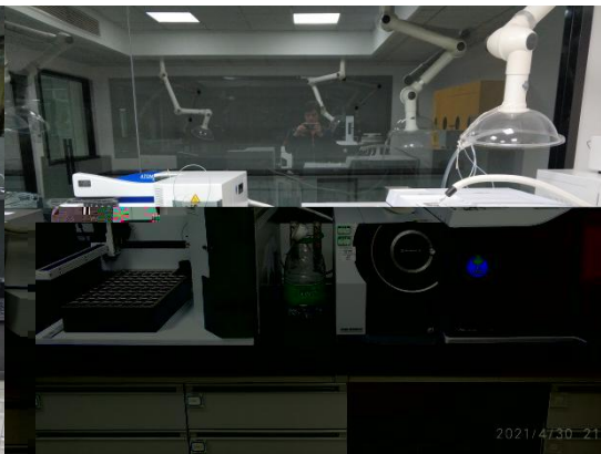
气相色谱与质谱联用仪-2
