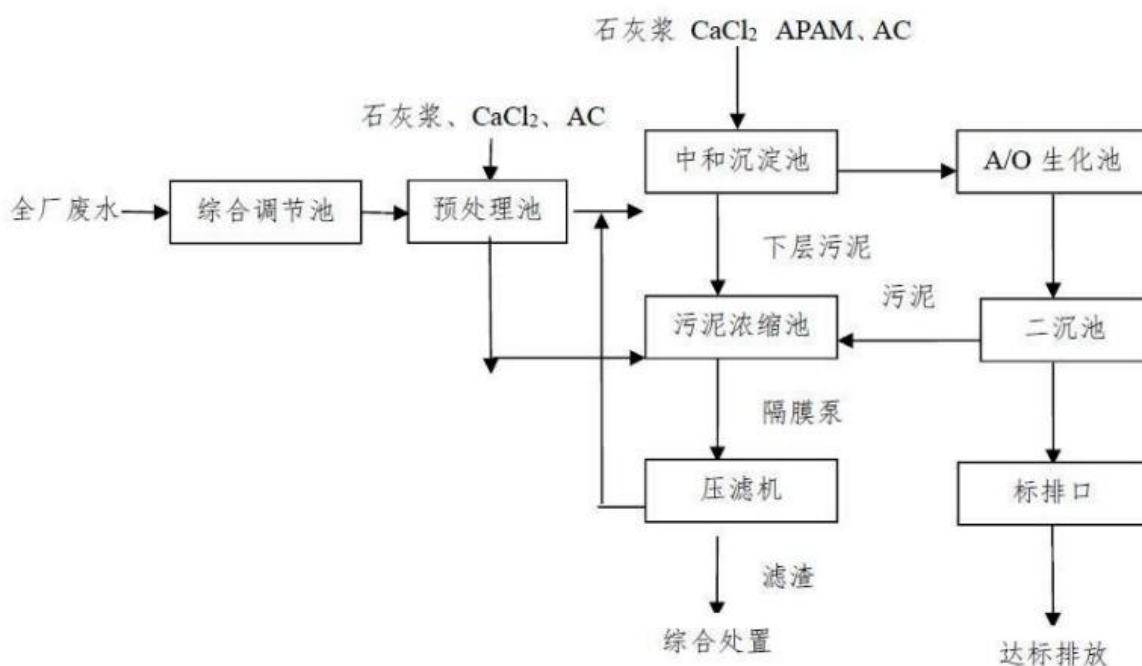
图 4.4.2-1 废水处理工艺流程图
